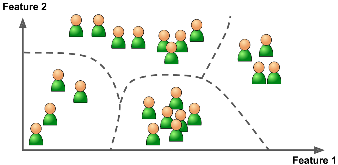
Figure 1-8. Clustering
