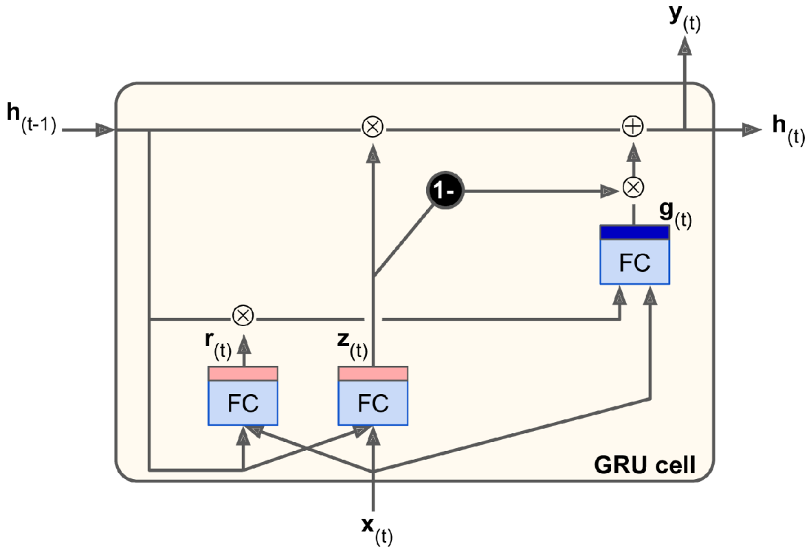
Figure 15-10. GRU cell
